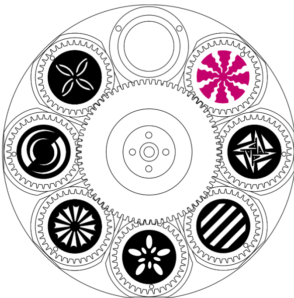
Rotierendes Goborad
